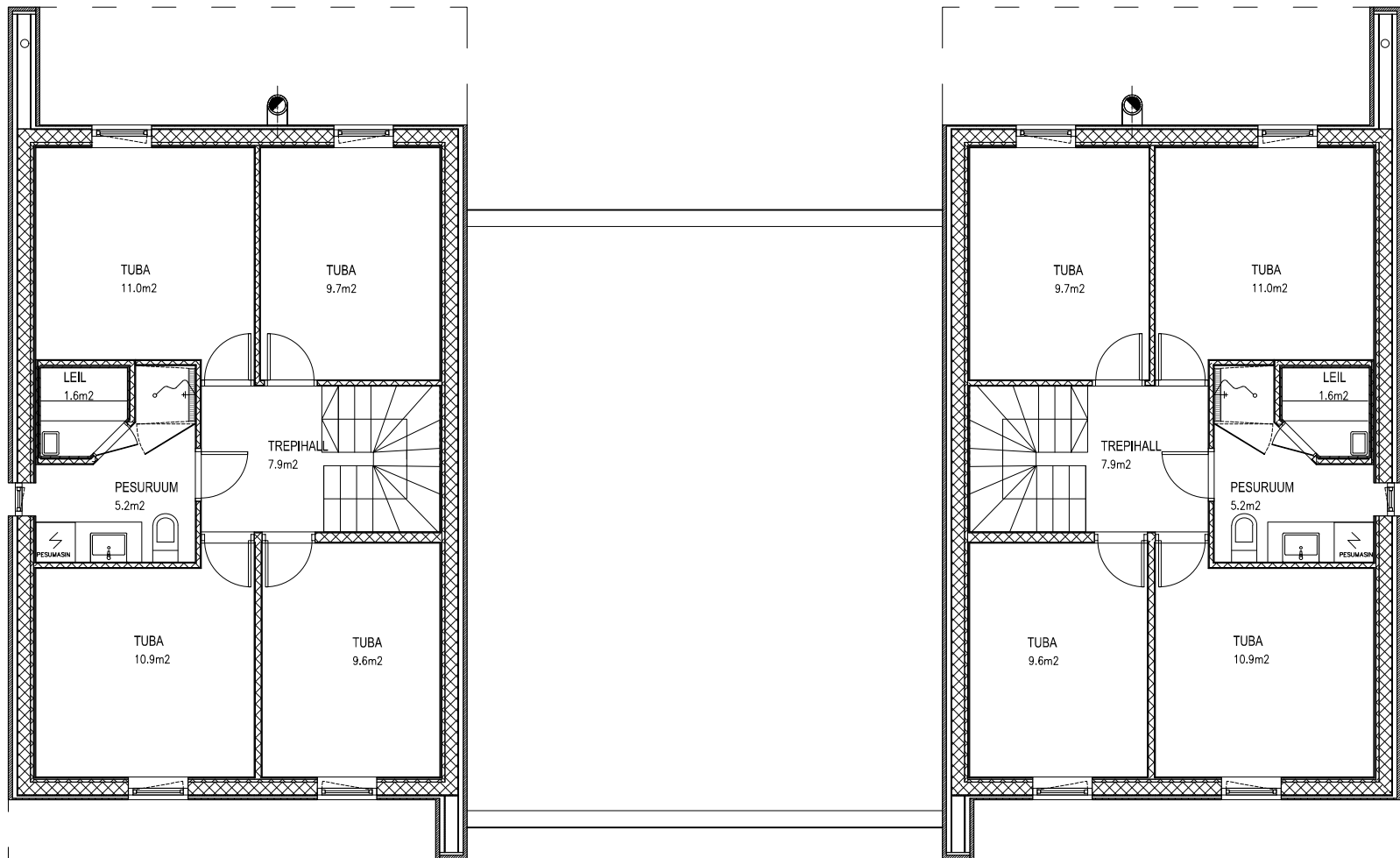
TEINE KORRUS
